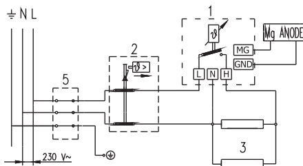
Электросхема
